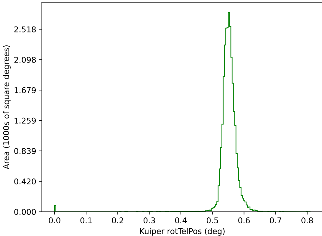
too_ignore_100_4v3.4_10yrs g: Kuiper rotTelPos
