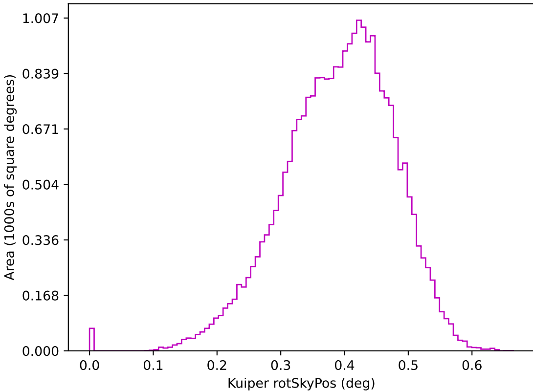
too_ignore_100_4v3.4_10yrs z: Kuiper rotSkyPos
