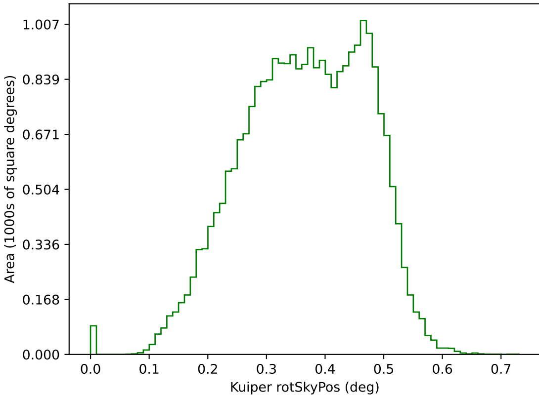
too_ignore_100_4v3.4_10yrs g: Kuiper rotSkyPos
