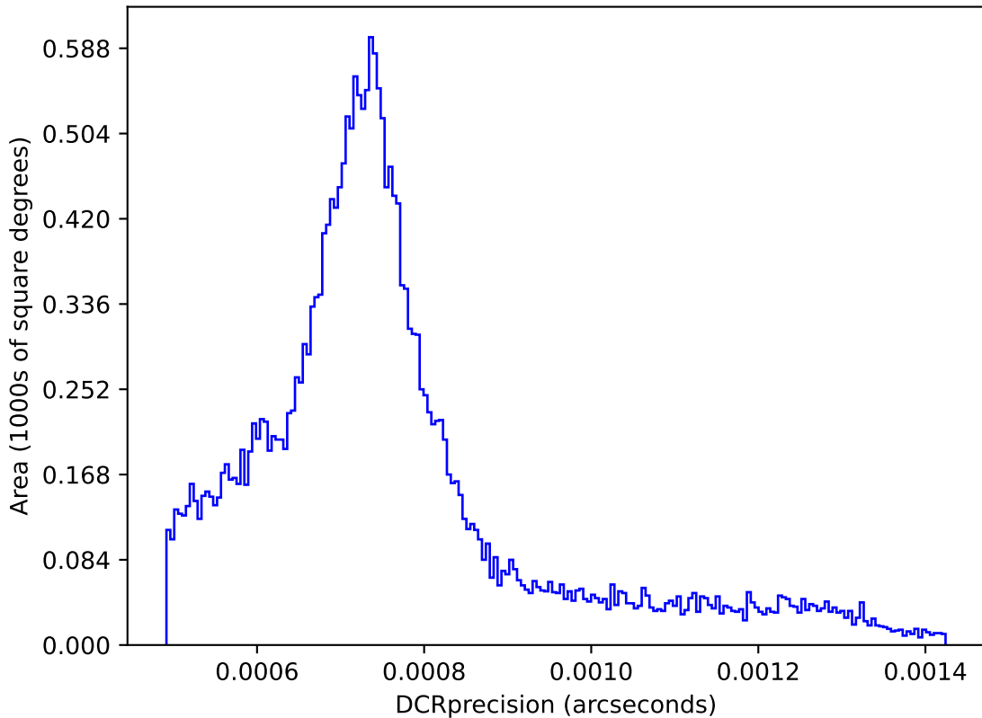
too_ignore_100_4v3.4_10yrs : DCRprecision
