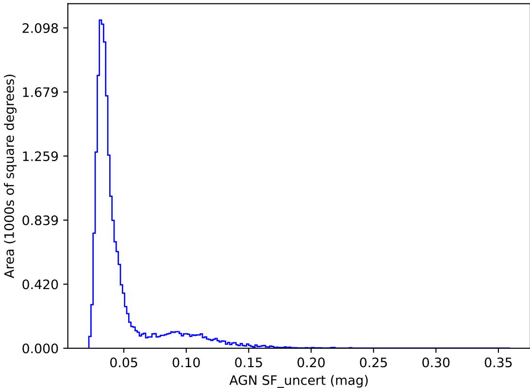
too_ignore_100_4v3.4_10yrs y band: AGN SF_uncert
