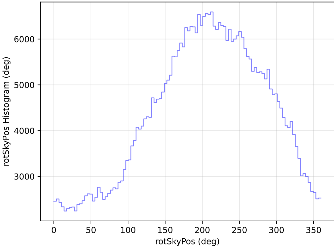
too_ignore_100_4v3.4_10yrs WFD z band: rotSkyPos Histogram
