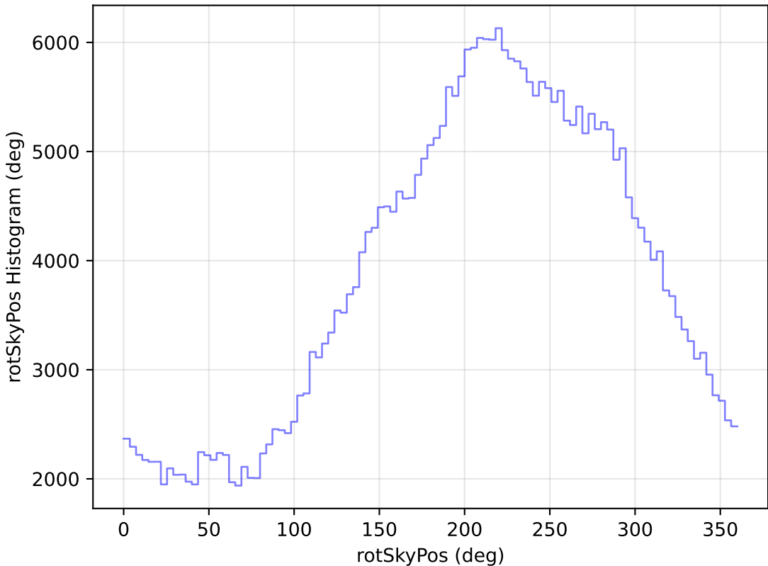
too_ignore_100_4v3.4_10yrs WFD y band: rotSkyPos Histogram
