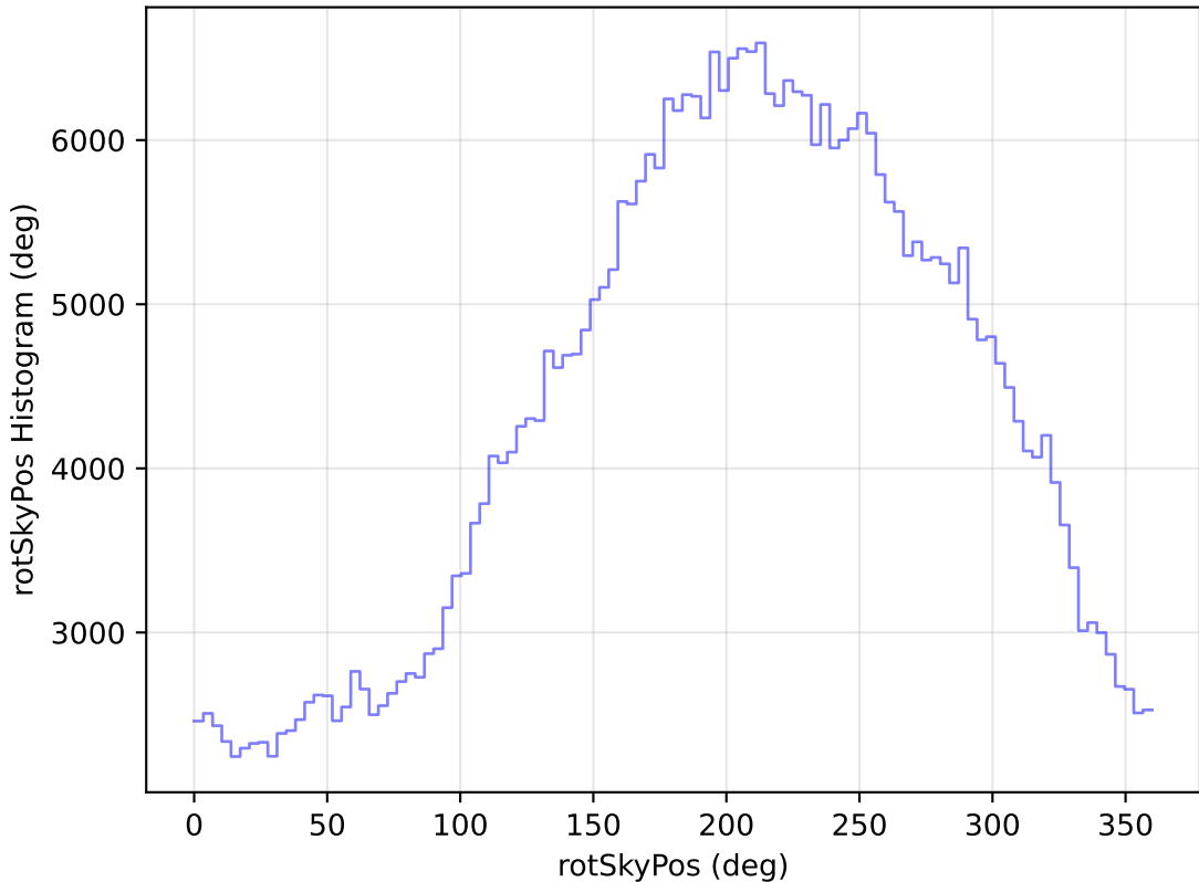
too_ignore_100_4v3.4_10yrs All sky z band: rotSkyPos Histogram
