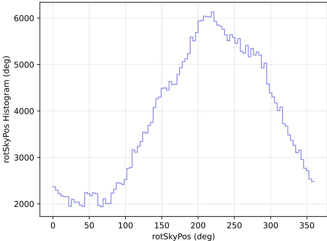
too_ignore_100_4v3.4_10yrs All sky y band: rotSkyPos Histogram
