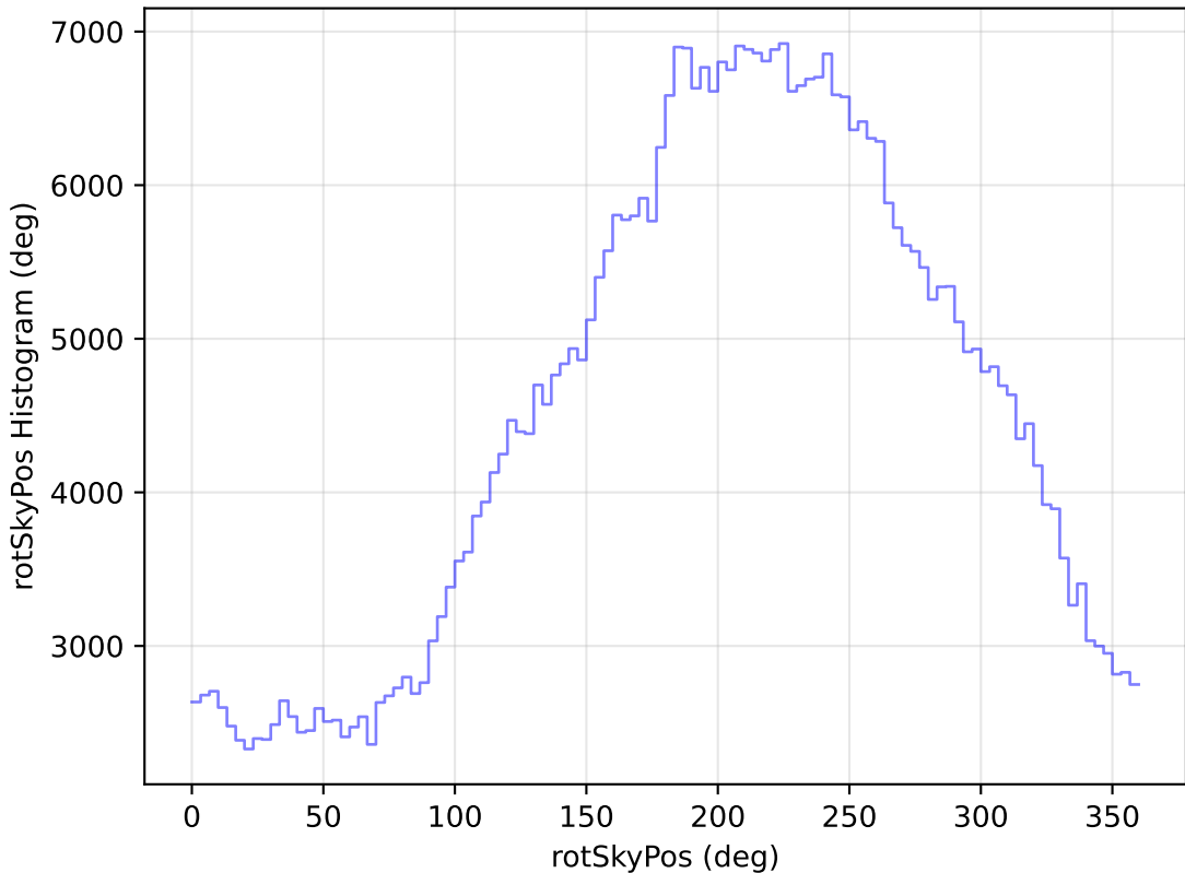
too_ignore_100_4v3.4_10yrs All sky i band: rotSkyPos Histogram
