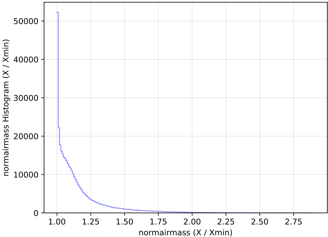
too_ignore_100_4v3.4_10yrs WFD y band: normairmass Histogram
