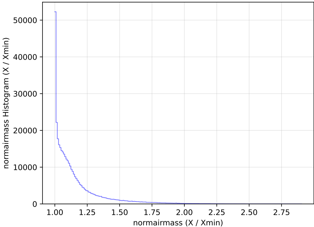
too_ignore_100_4v3.4_10yrs All sky y band: normairmass Histogram
