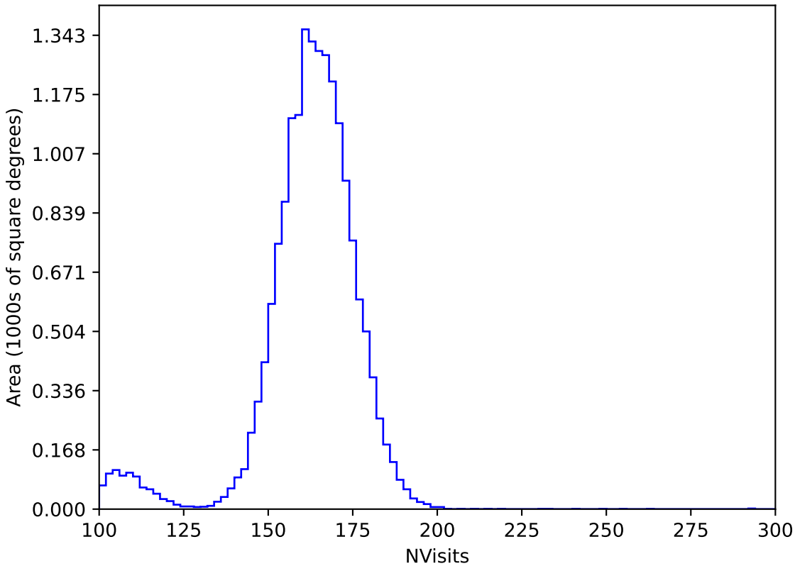
too_ignore_100_4v3.4_10yrs WFD y band: NVisits
