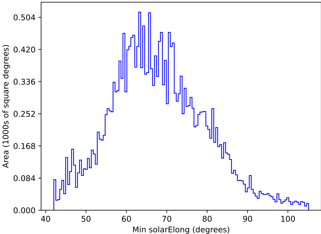
too_ignore_100_4v3.4_10yrs All sky y band: Min solarElong
