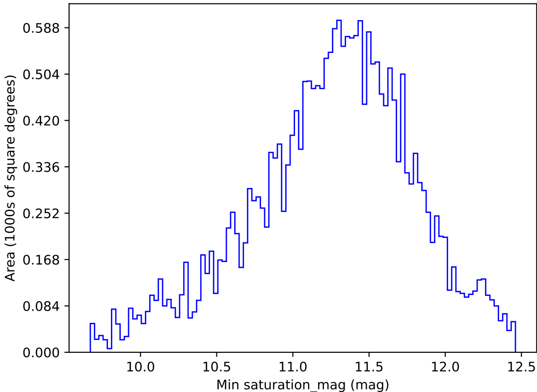
too_ignore_100_4v3.4_10yrs All sky y band: Min saturation_mag
