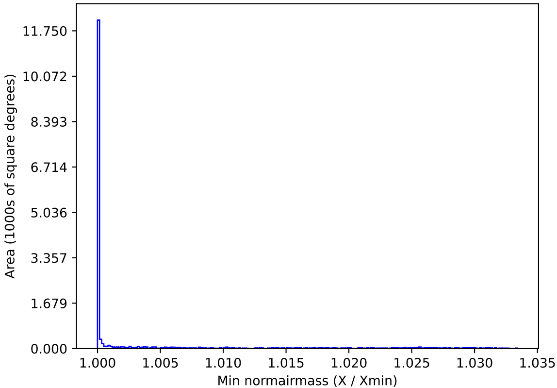
too_ignore_100_4v3.4_10yrs WFD z band: Min normairmass
