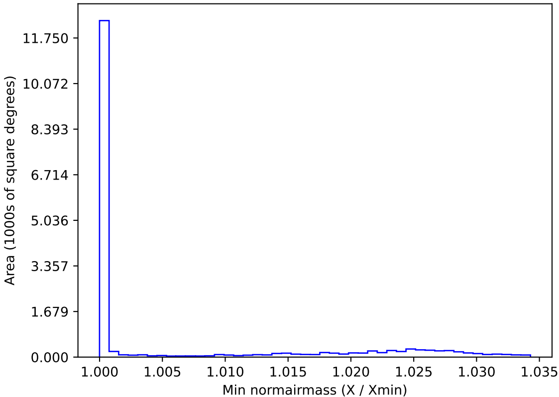
too_ignore_100_4v3.4_10yrs WFD i band: Min normairmass
