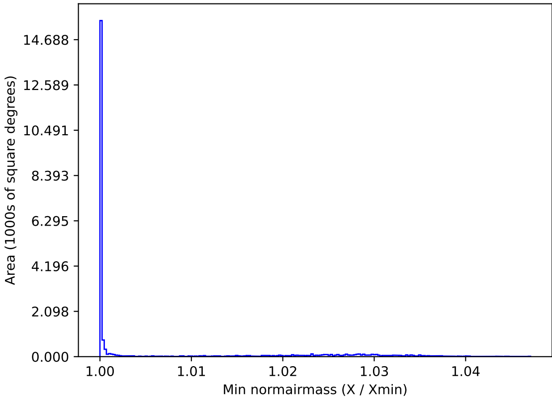
too_ignore_100_4v3.4_10yrs All sky y band: Min normairmass
