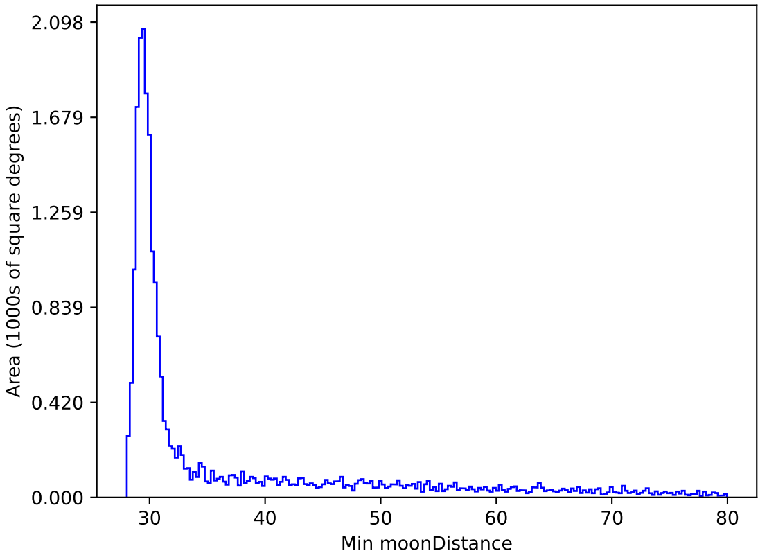
too_ignore_100_4v3.4_10yrs All sky y band: Min moonDistance
