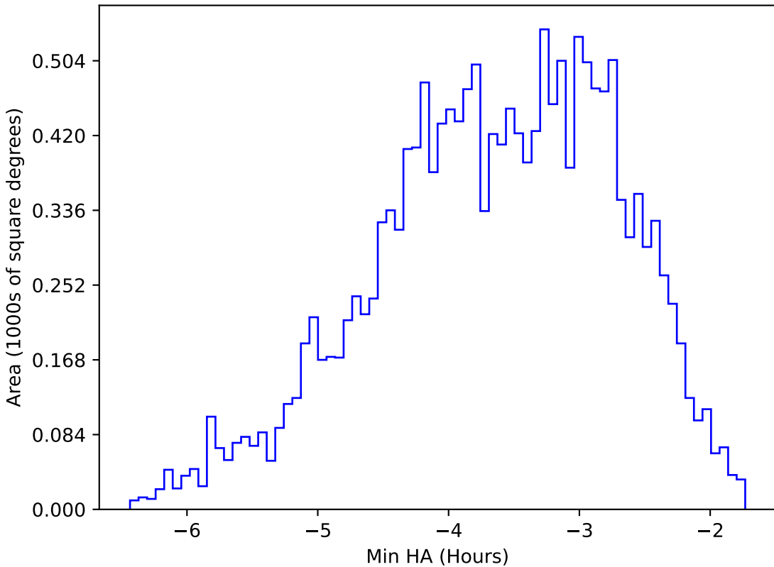
too_ignore_100_4v3.4_10yrs WFD y band: Min HA
