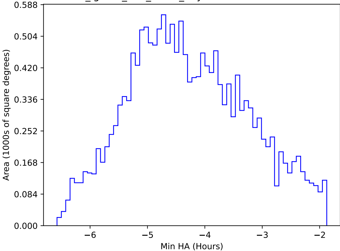
too_ignore_100_4v3.4_10yrs WFD i band: Min HA
