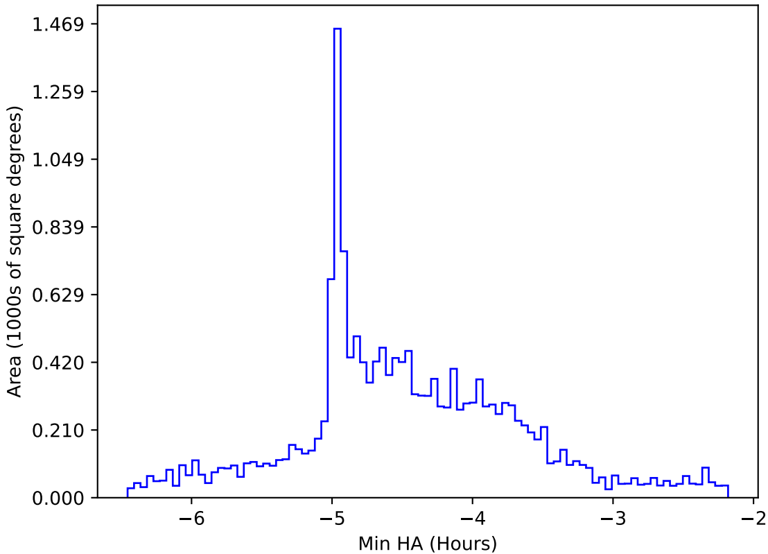
too_ignore_100_4v3.4_10yrs WFD g band: Min HA
