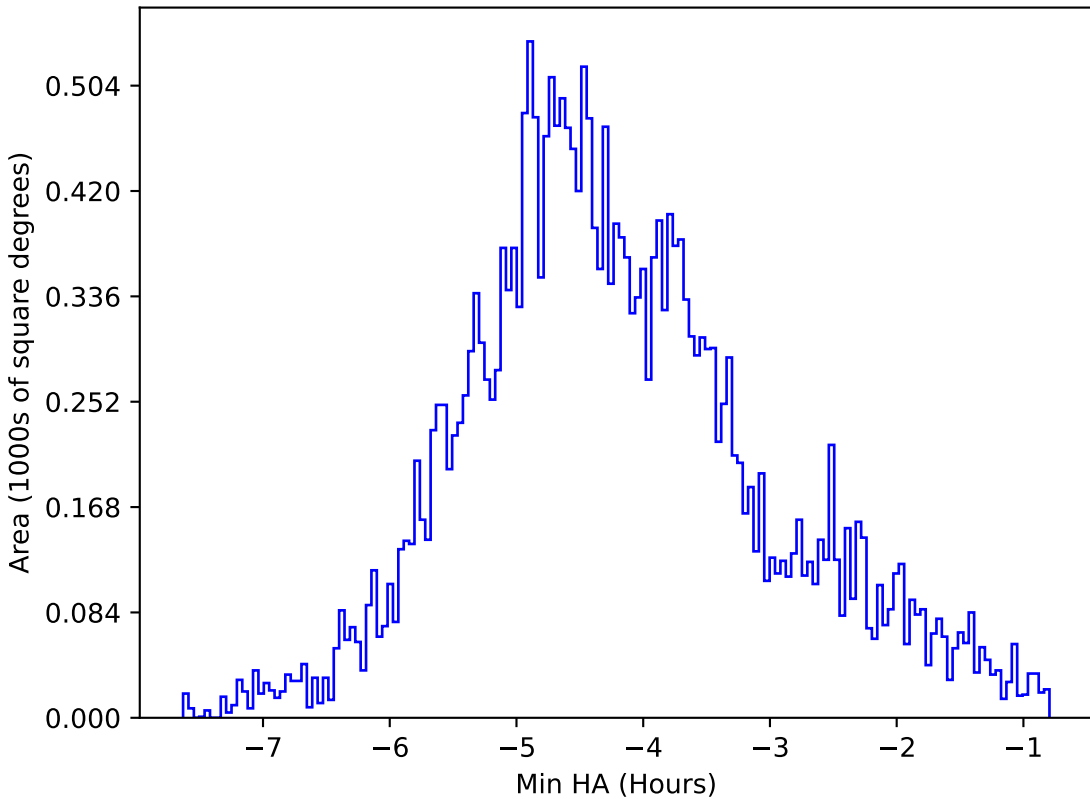
too_ignore_100_4v3.4_10yrs All sky z band: Min HA
