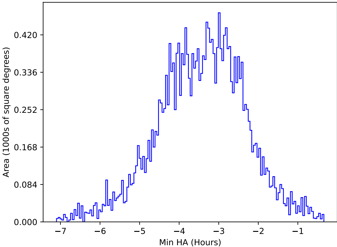
too_ignore_100_4v3.4_10yrs All sky y band: Min HA
