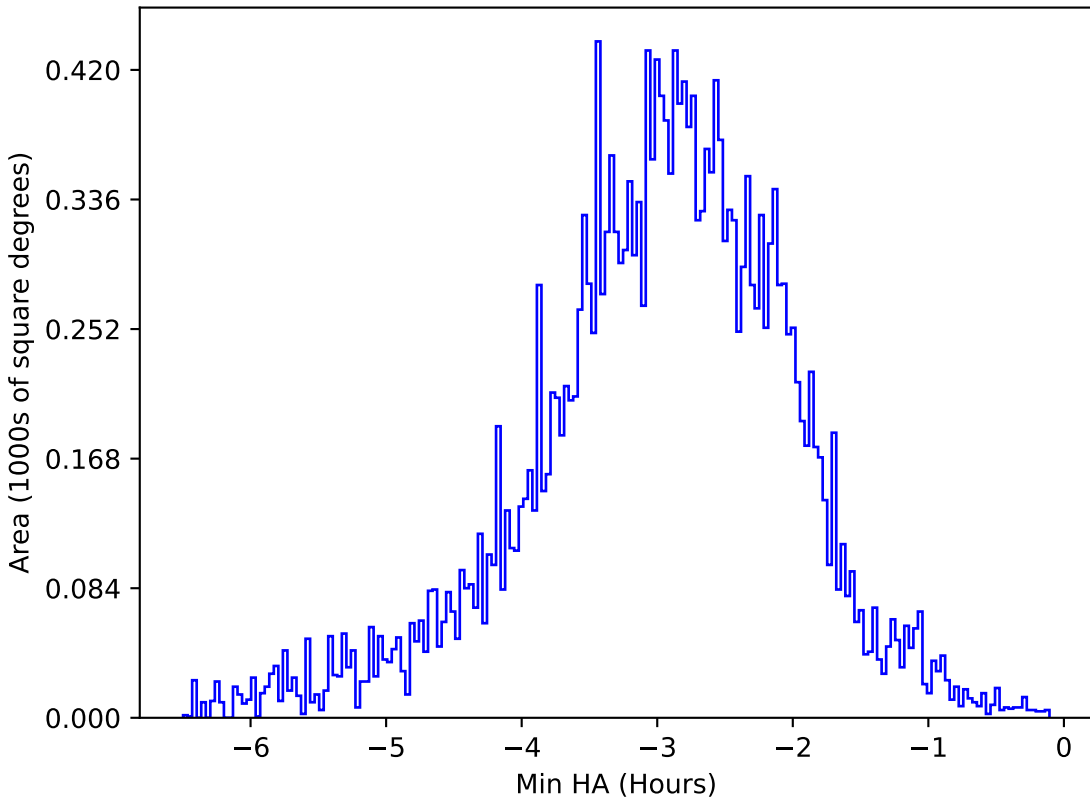
too_ignore_100_4v3.4_10yrs All sky u band: Min HA
