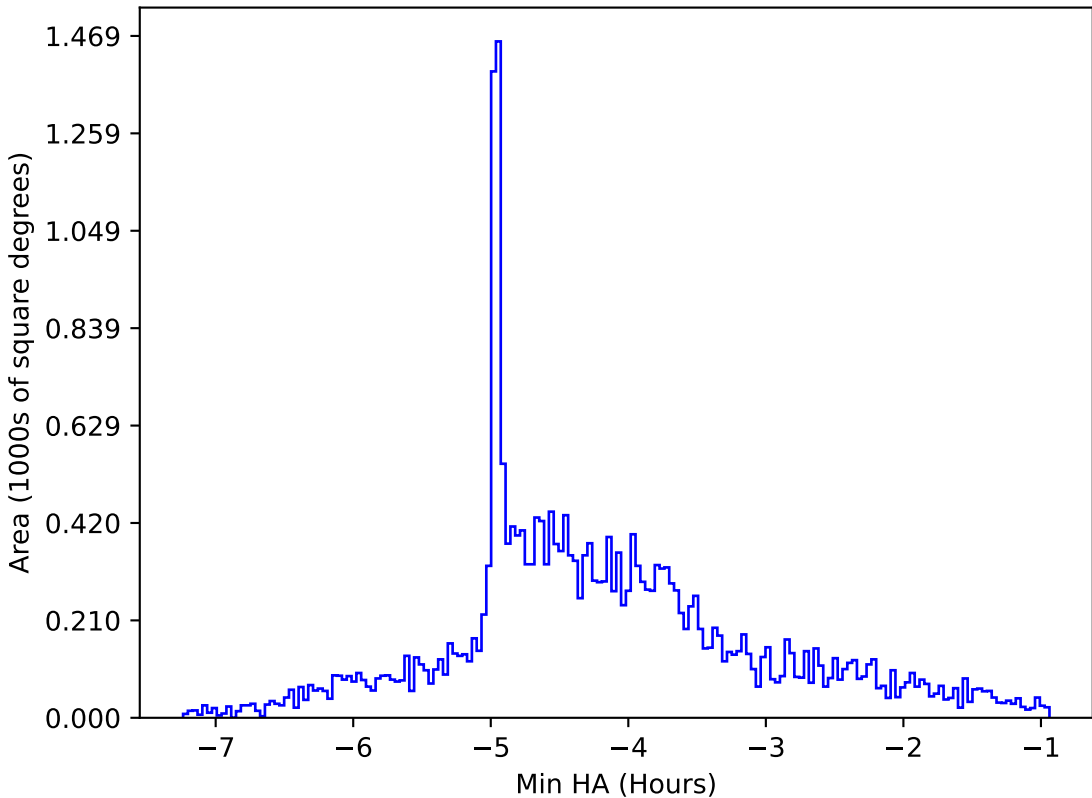
too_ignore_100_4v3.4_10yrs All sky g band: Min HA
