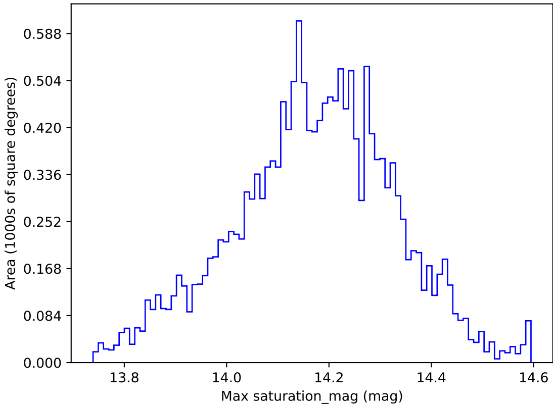
too_ignore_100_4v3.4_10yrs WFD y band: Max saturation_mag
