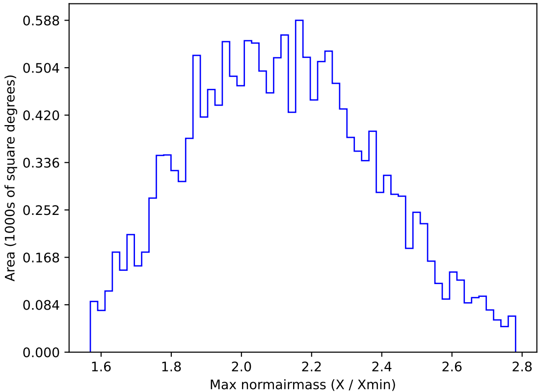
too_ignore_100_4v3.4_10yrs WFD y band: Max normairmass
