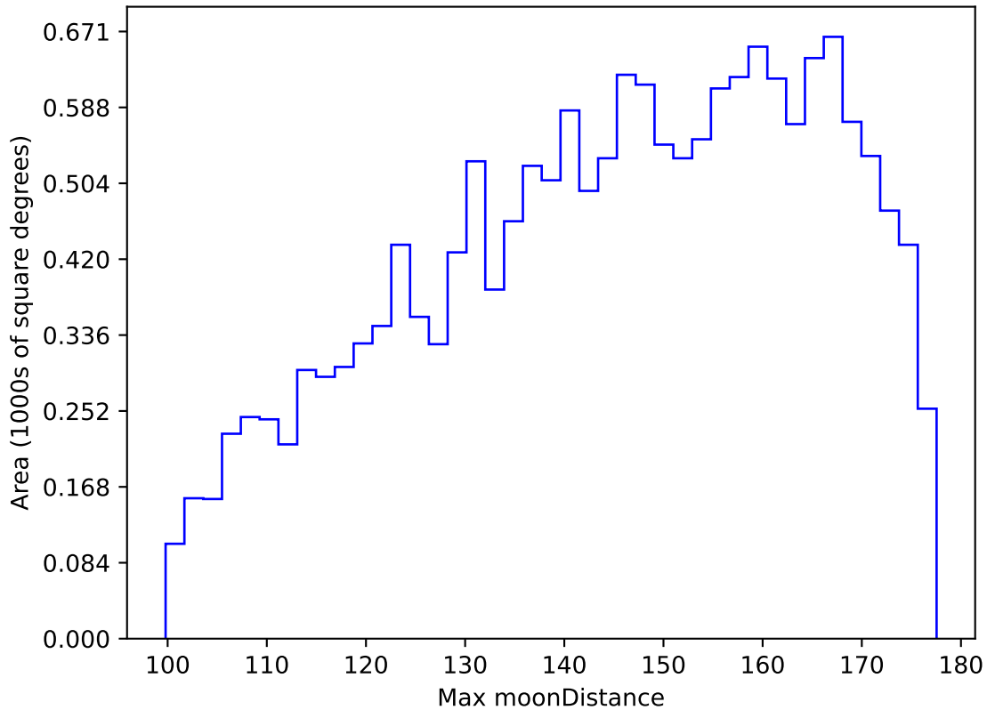
too_ignore_100_4v3.4_10yrs WFD y band: Max moonDistance
