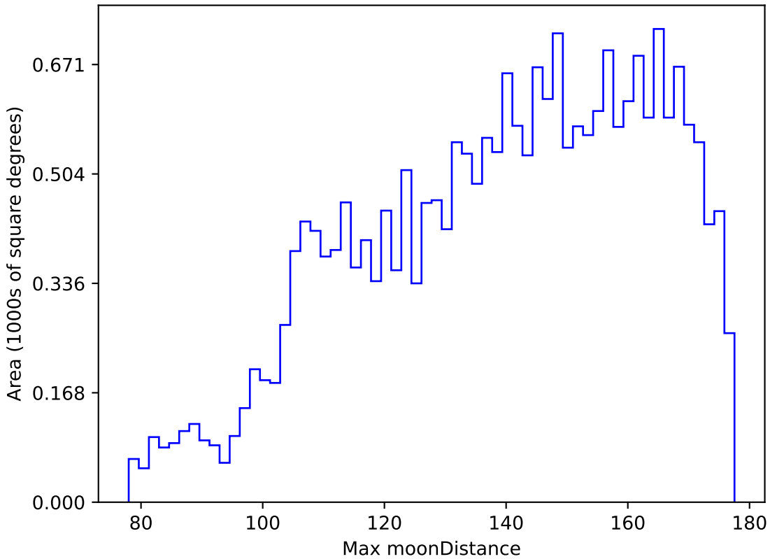
too_ignore_100_4v3.4_10yrs All sky y band: Max moonDistance
