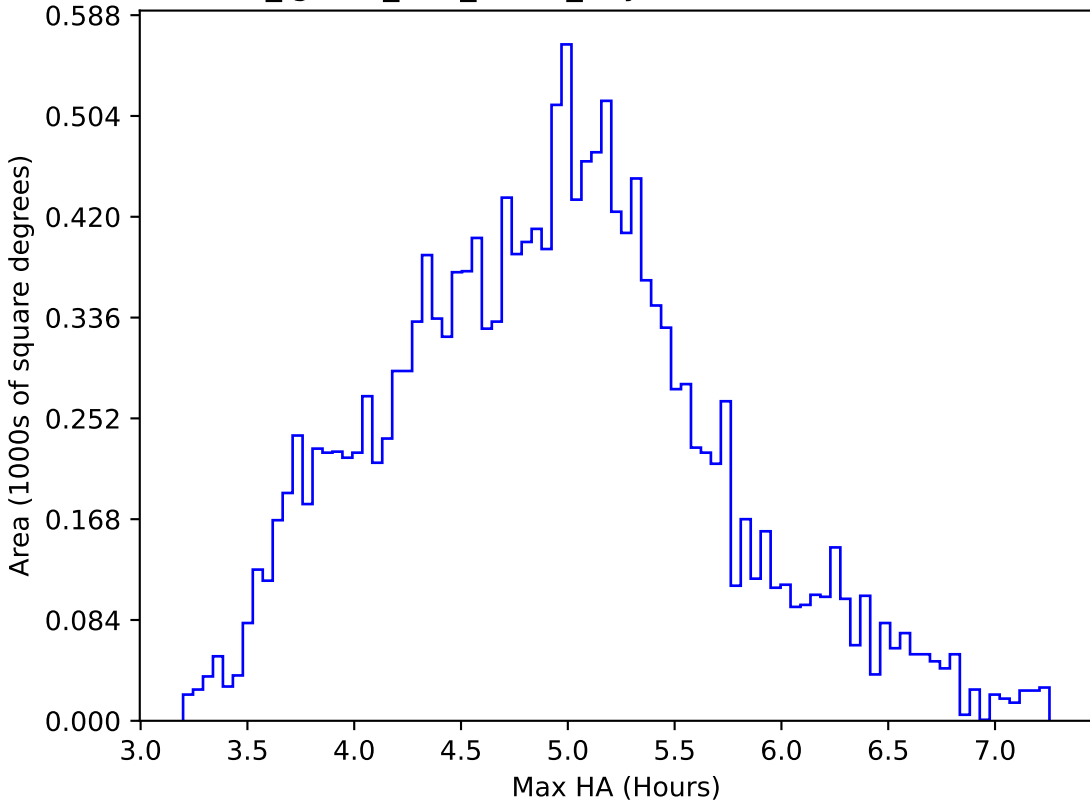
too_ignore_100_4v3.4_10yrs WFD z band: Max HA
