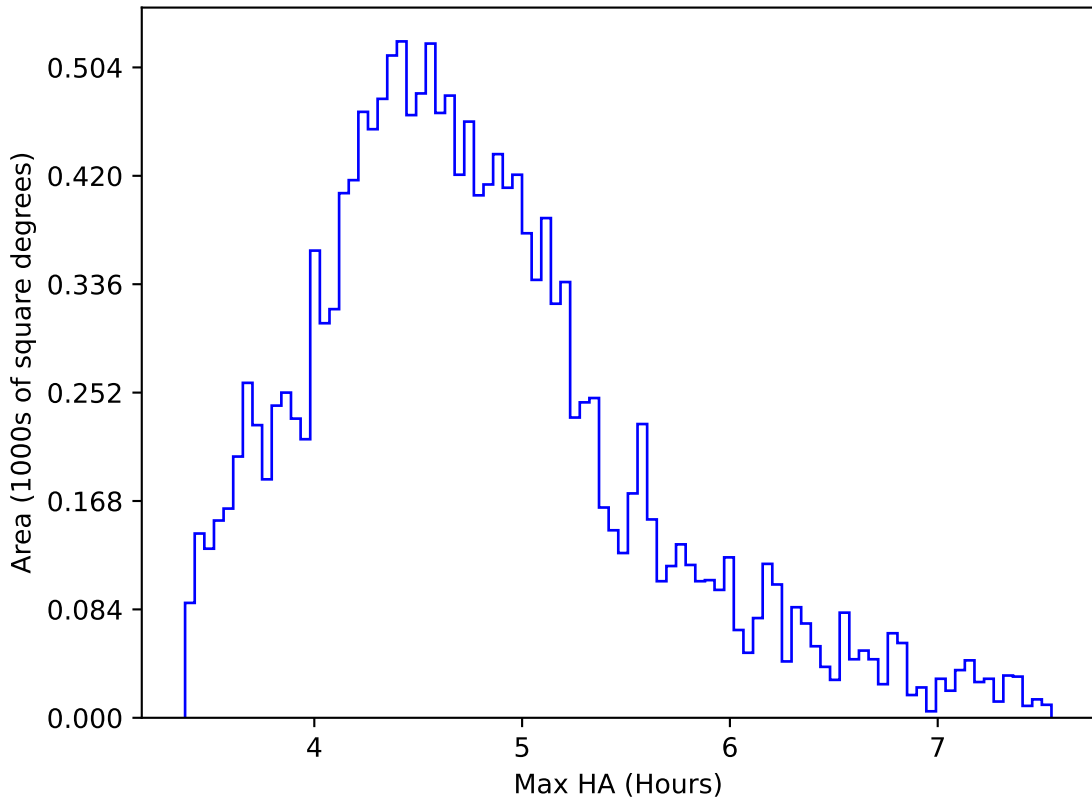
too_ignore_100_4v3.4_10yrs WFD y band: Max HA
