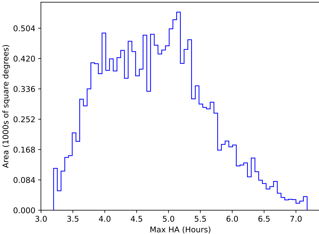
too_ignore_100_4v3.4_10yrs WFD i band: Max HA
