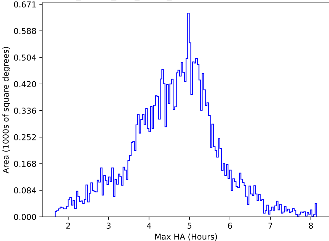
too_ignore_100_4v3.4_10yrs All sky z band: Max HA
