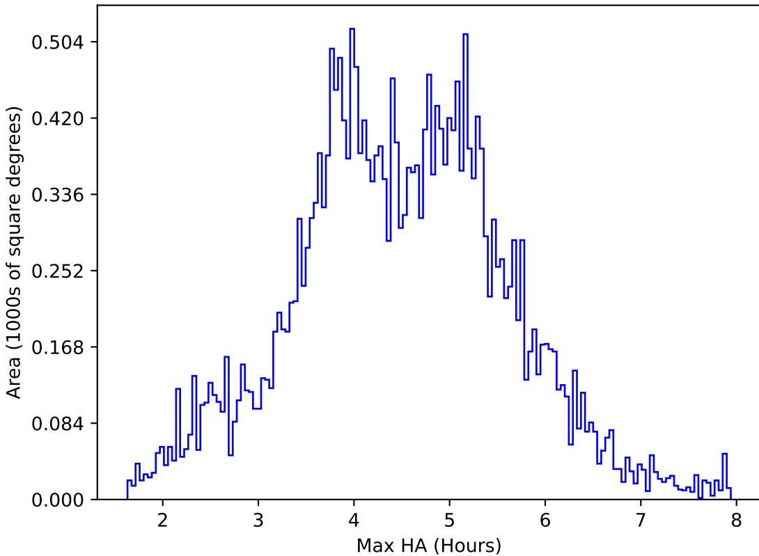
too_ignore_100_4v3.4_10yrs All sky i band: Max HA
