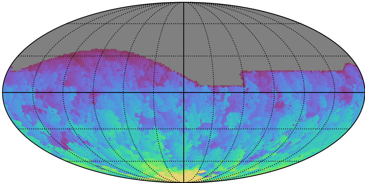
too_ignore_100_4v3.4_10yrs All sky g band: Max HA
