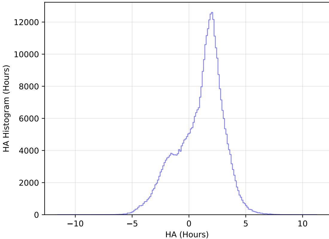
too_ignore_100_4v3.4_10yrs WFD y band: HA Histogram
