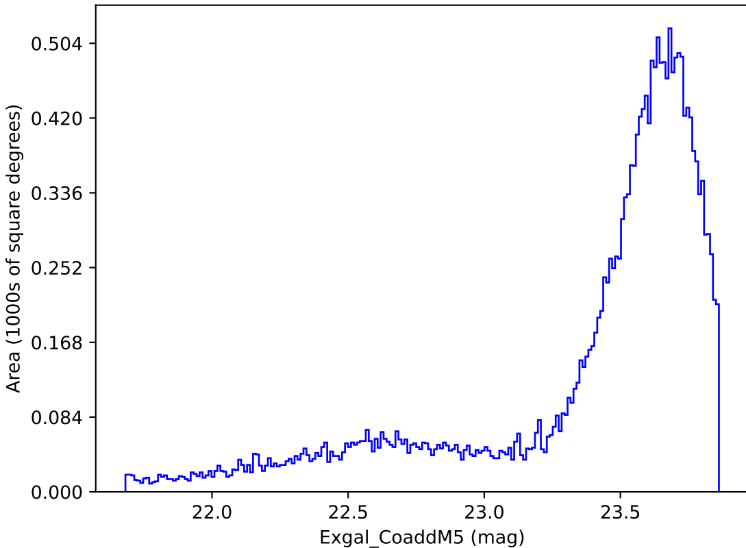
too_ignore_100_4v3.4_10yrs Yr 1 y band: Exgal_CoaddM5
