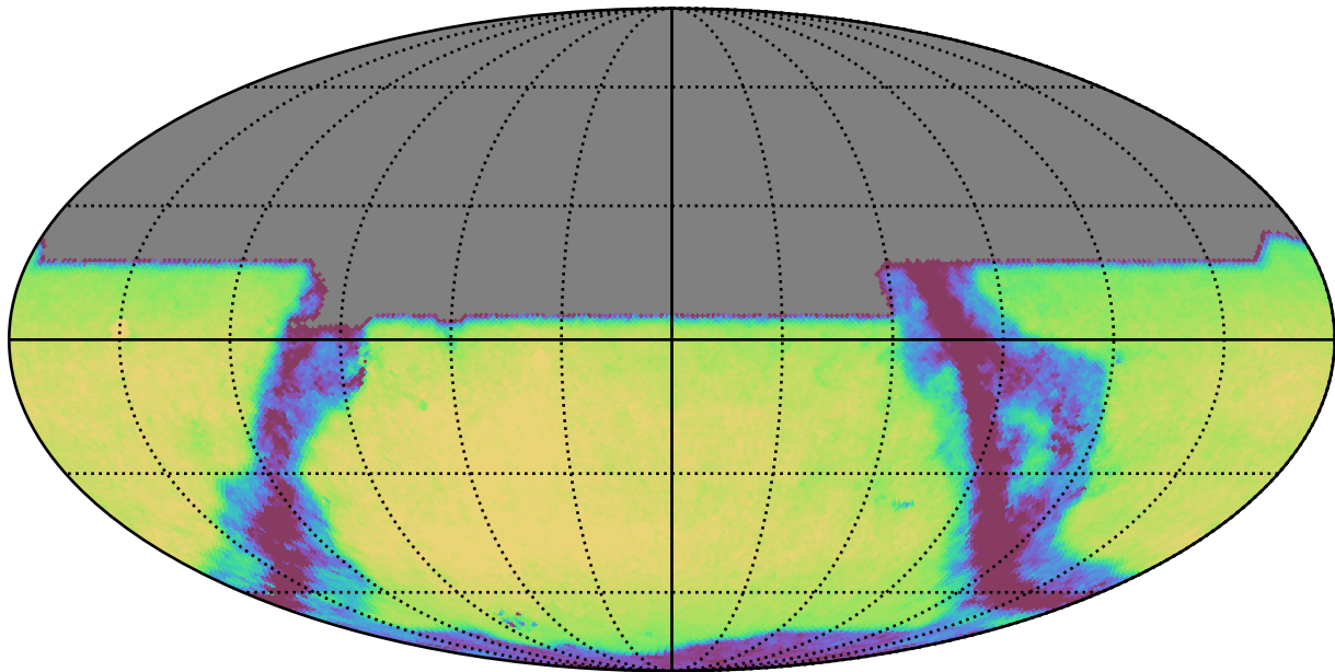
too_ignore_100_4v3.4_10yrs All sky y band: Exgal_CoaddM5
