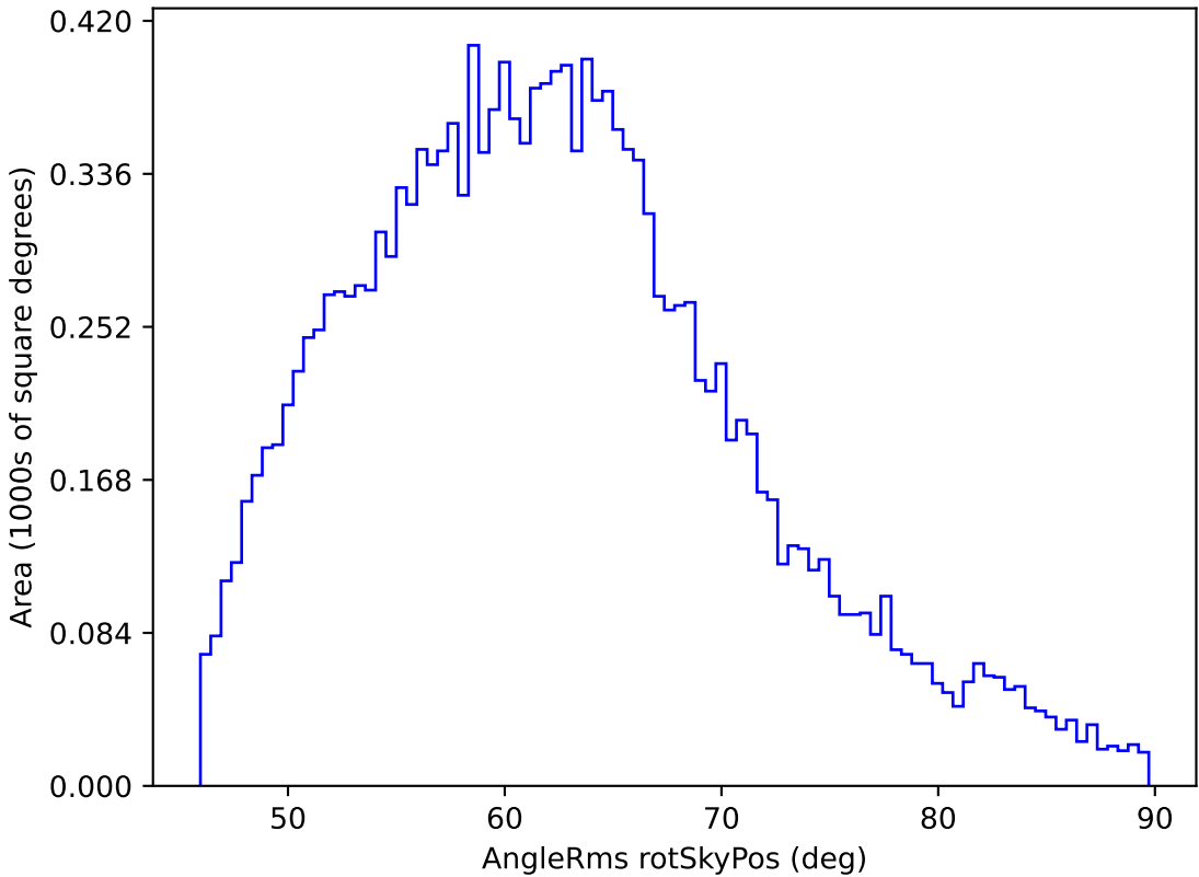
too_ignore_100_4v3.4_10yrs WFD y band: AngleRms rotSkyPos
