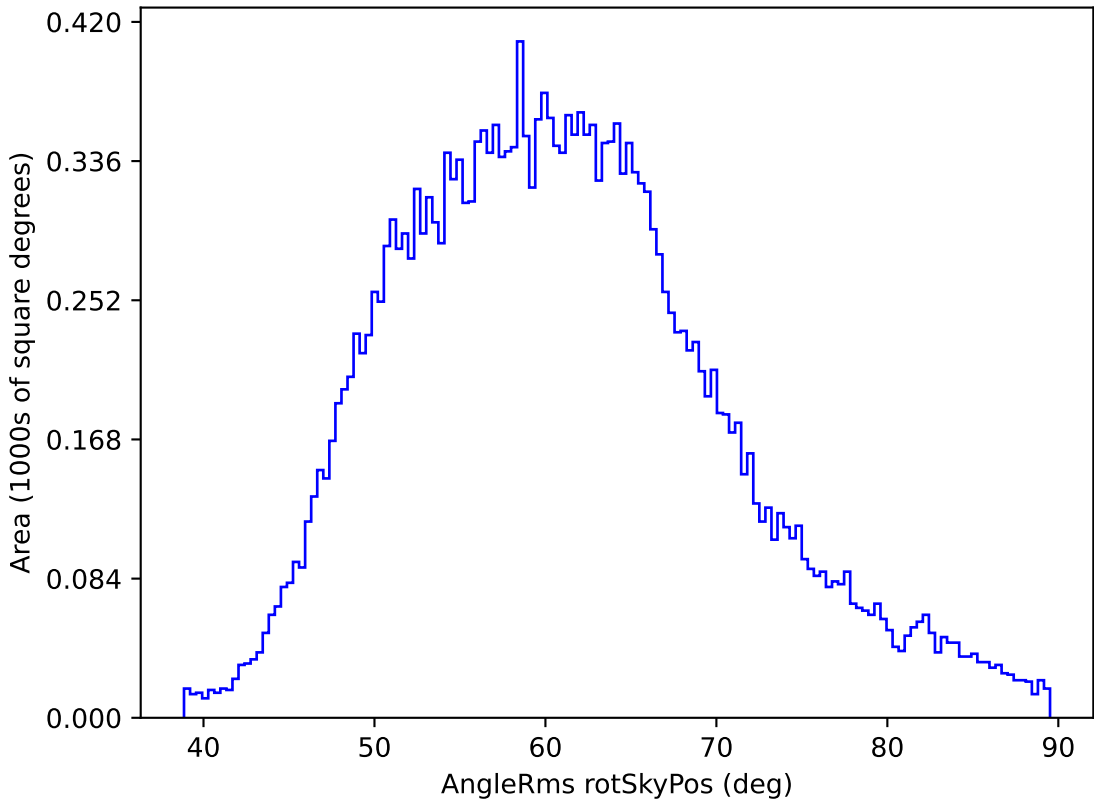
too_ignore_100_4v3.4_10yrs All sky y band: AngleRms rotSkyPos
