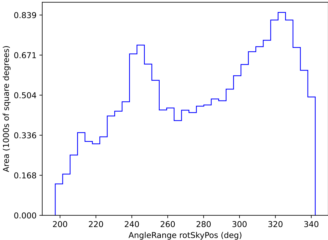
too_ignore_100_4v3.4_10yrs WFD z band: AngleRange rotSkyPos
