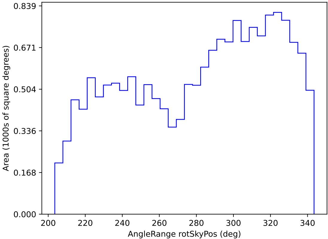
too_ignore_100_4v3.4_10yrs WFD r band: AngleRange rotSkyPos
