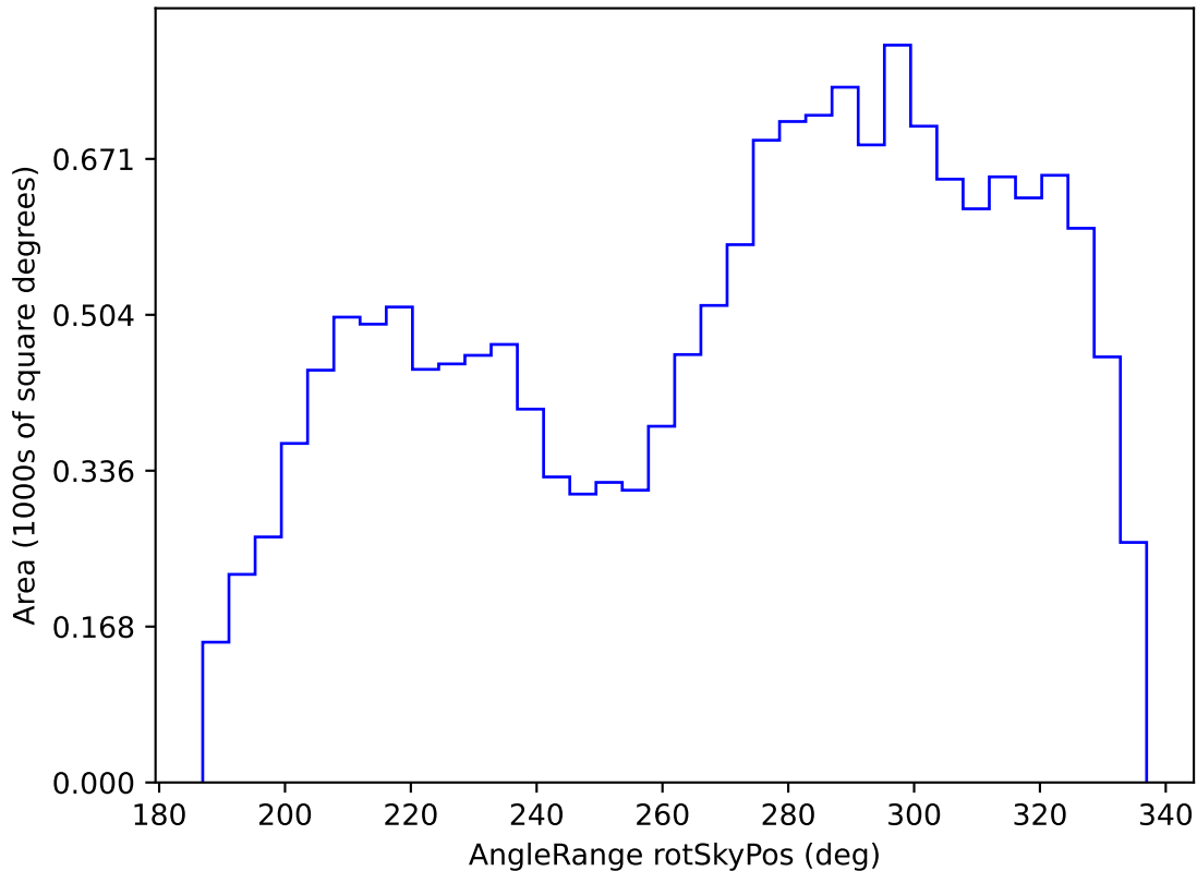
too_ignore_100_4v3.4_10yrs WFD g band: AngleRange rotSkyPos
