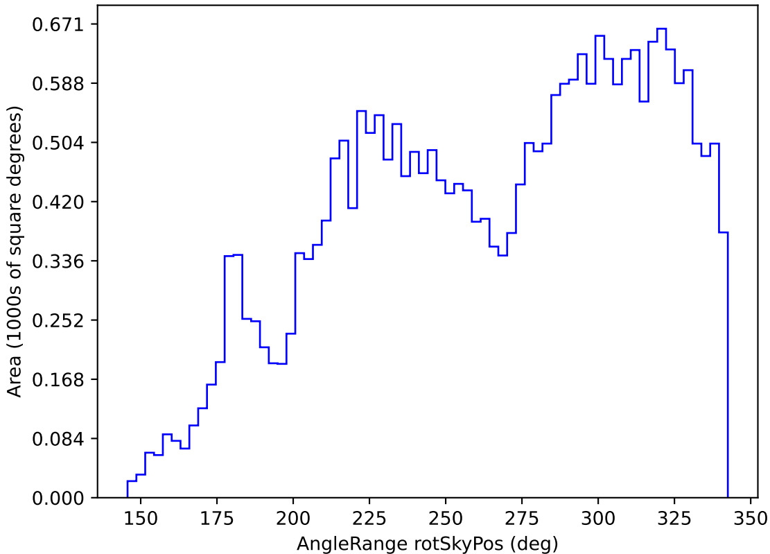
too_ignore_100_4v3.4_10yrs All sky r band: AngleRange rotSkyPos
