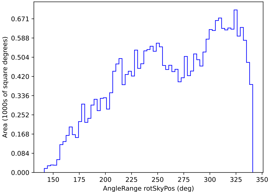
too_ignore_100_4v3.4_10yrs All sky i band: AngleRange rotSkyPos
