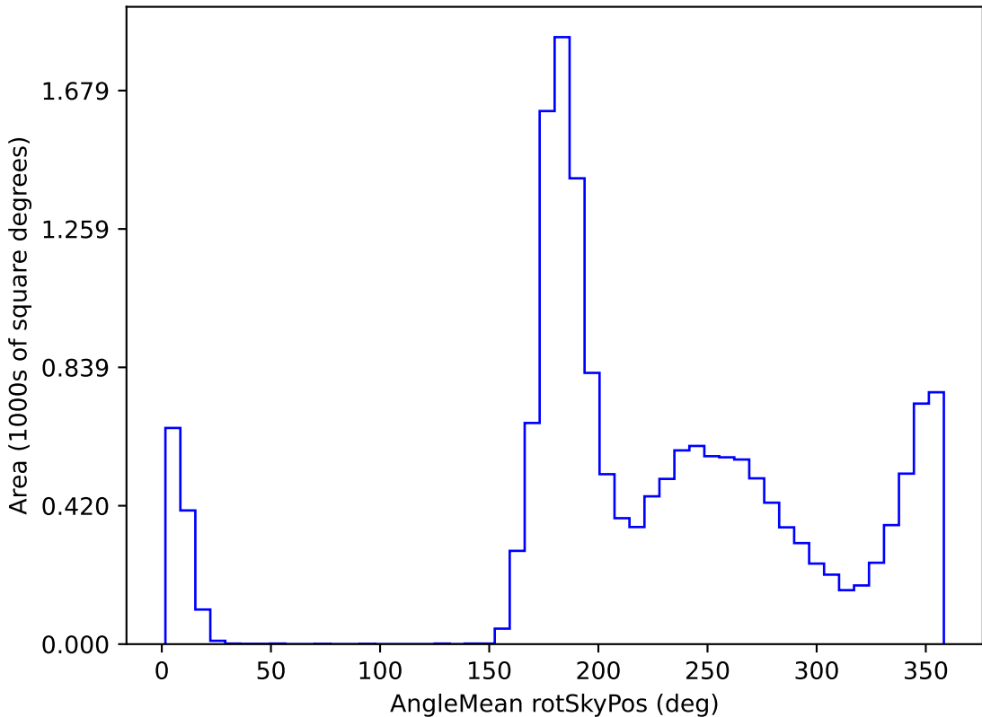
too_ignore_100_4v3.4_10yrs WFD y band: AngleMean rotSkyPos
