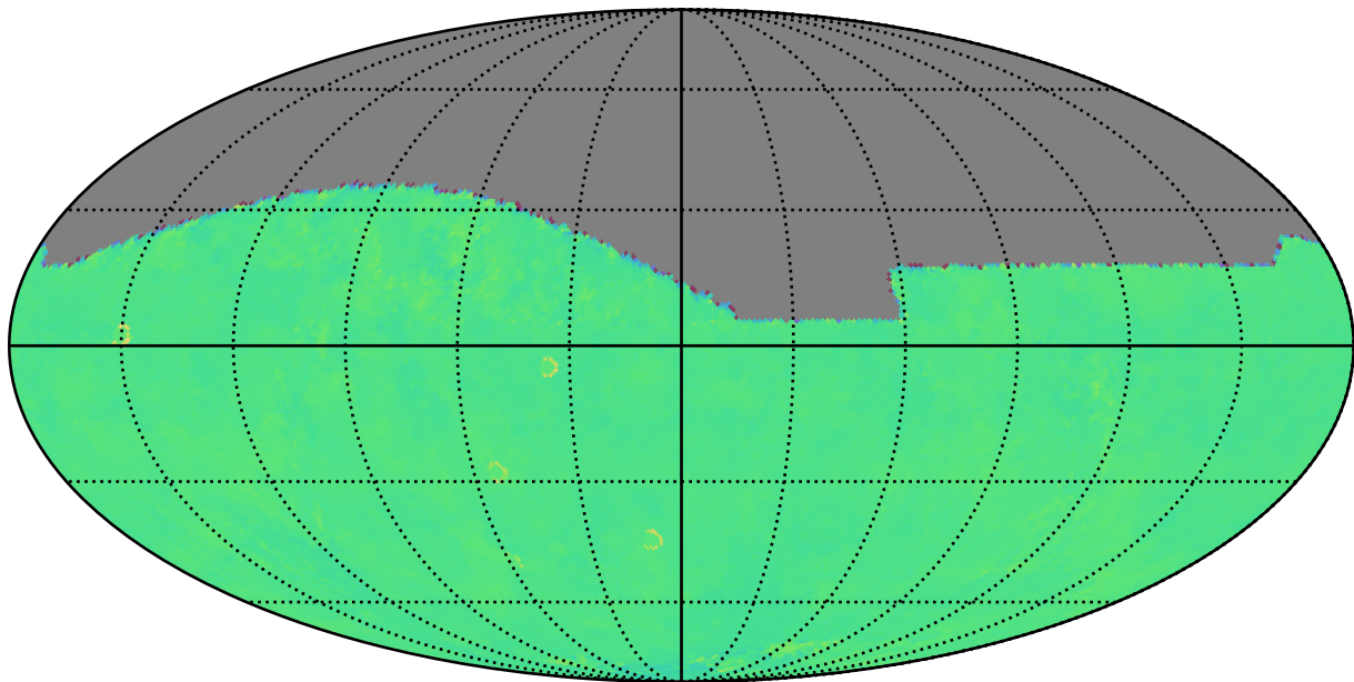
too_ignore_100_1v3.4_10yrs z: Kuiper rotTelPos
