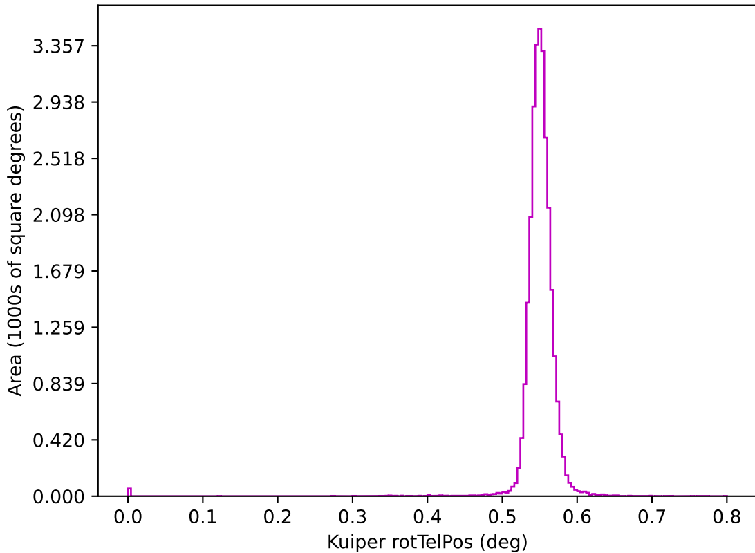
too_ignore_100_1v3.4_10yrs z: Kuiper rotTelPos
