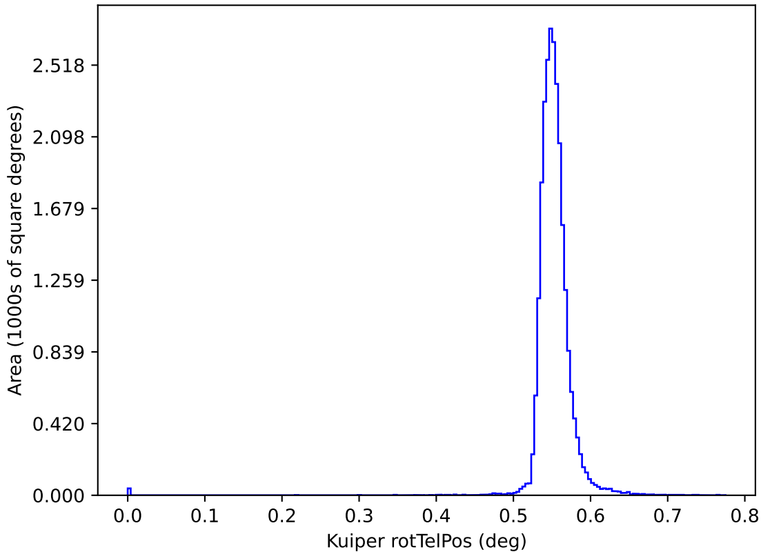
too_ignore_100_1v3.4_10yrs y: Kuiper rotTelPos
